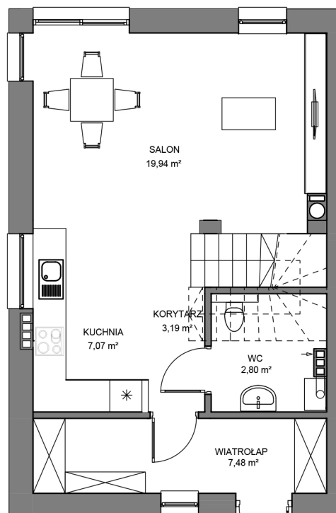
RZUT PARTERU
